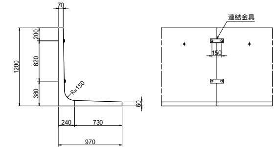
構造図
