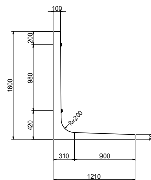
構造図
