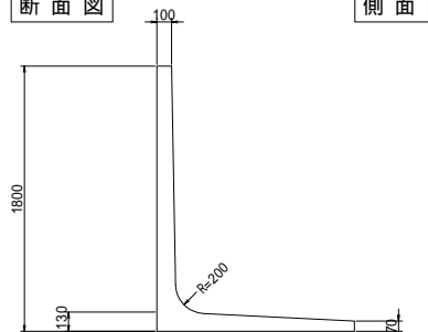
断面図
