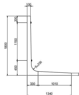
構造図
