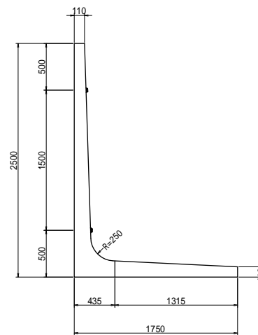
構造図
