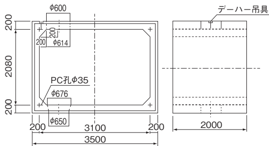
Cタイプ (底設・吸管取付部材)
