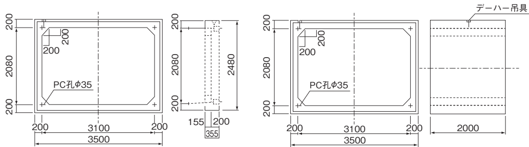
Aタイプ (端面部材)
