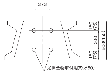
600 B・600 C・600 D (片面斜壁)
