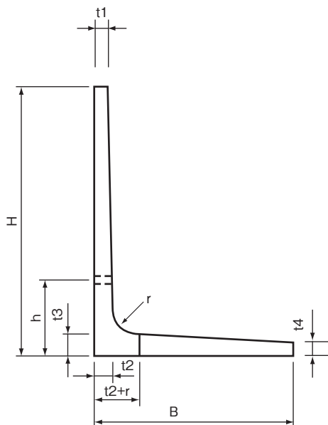
側面図
