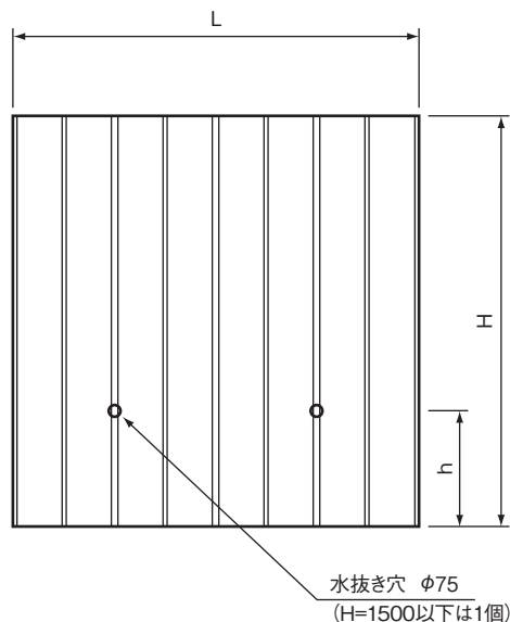
正面図
