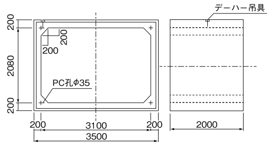
Bタイプ (中間部材)
