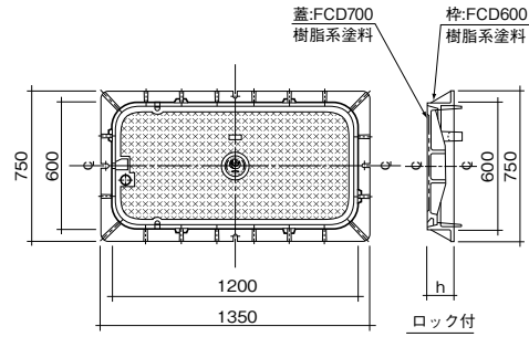
蓋 1,200×600詳細図
