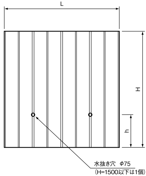
正面図
