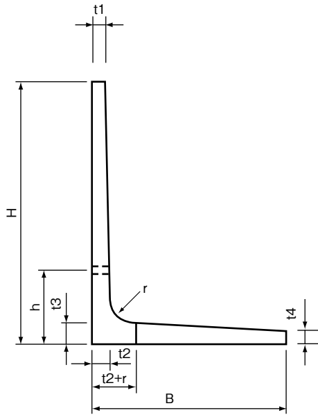
側面図
